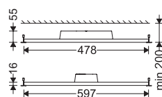
M528LED...
