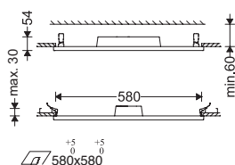
M528LED...+DMRC-15
